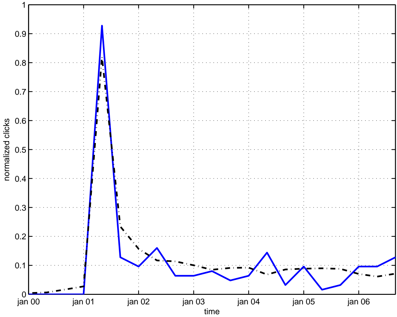
nonrenormalizable
