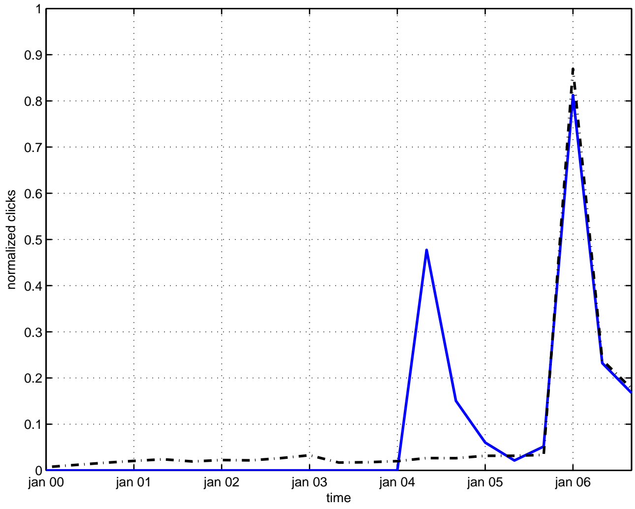
nonabelian vortex
