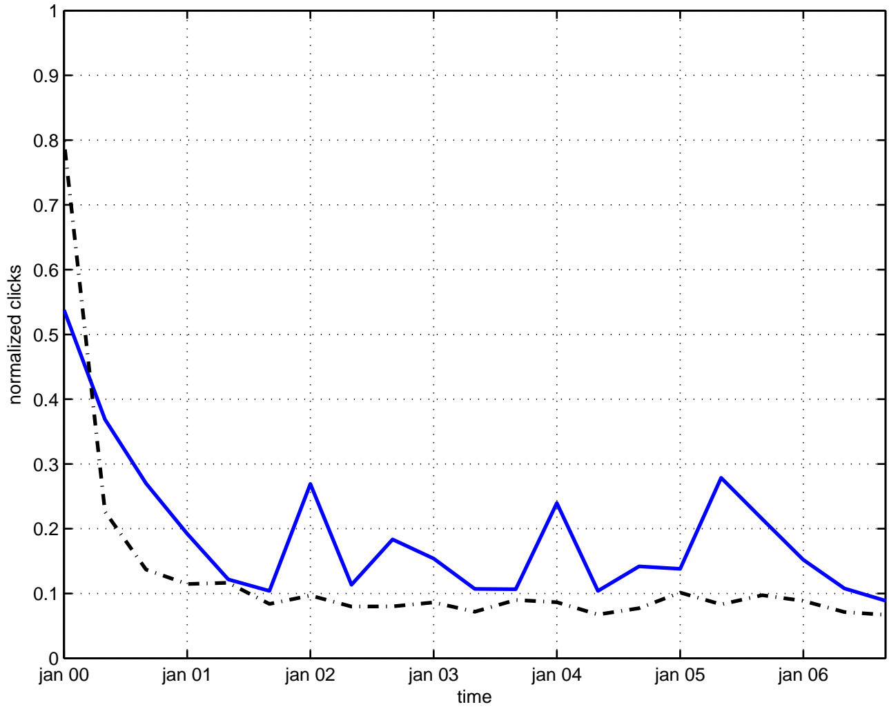
neutrino
