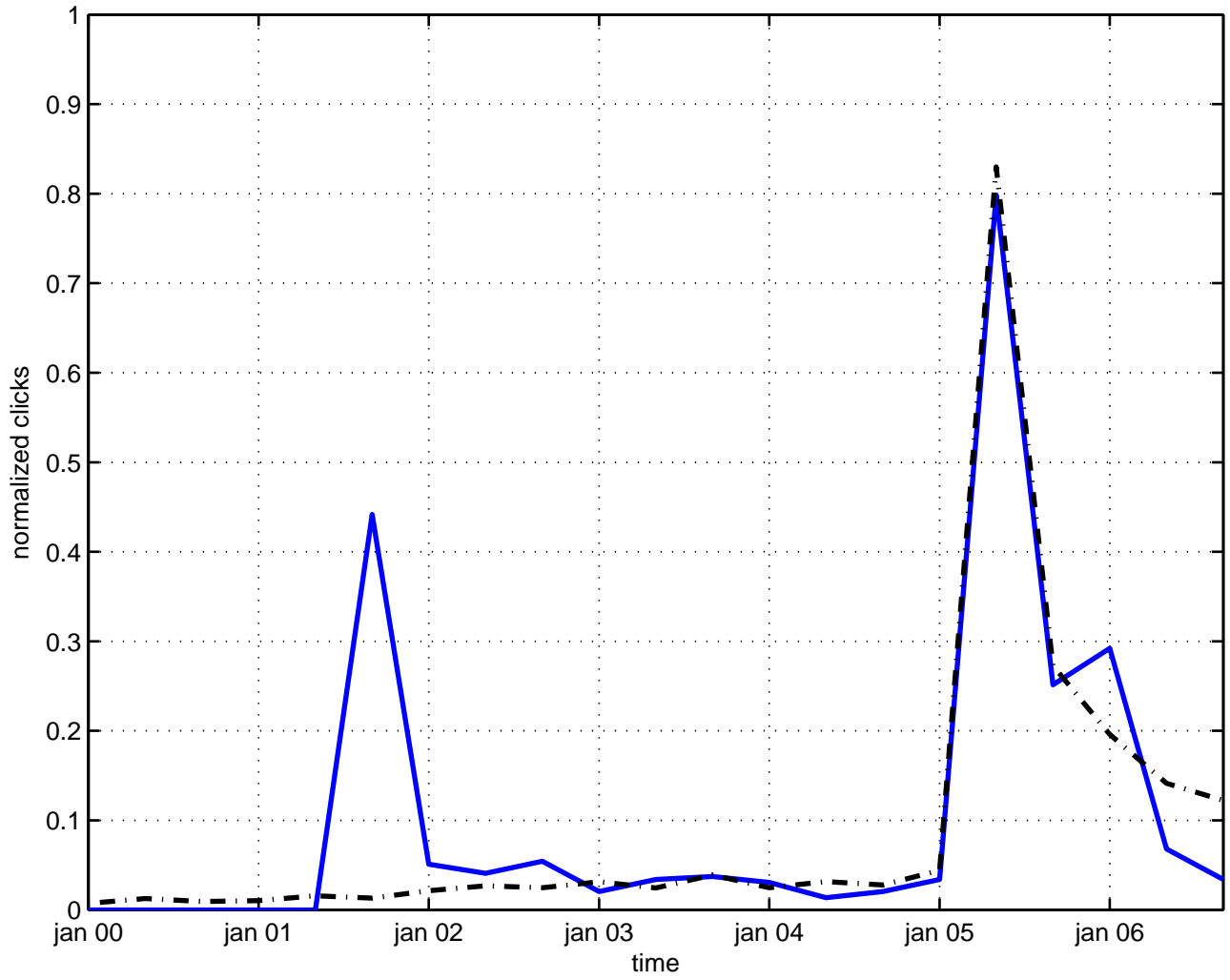
nariai black hole
