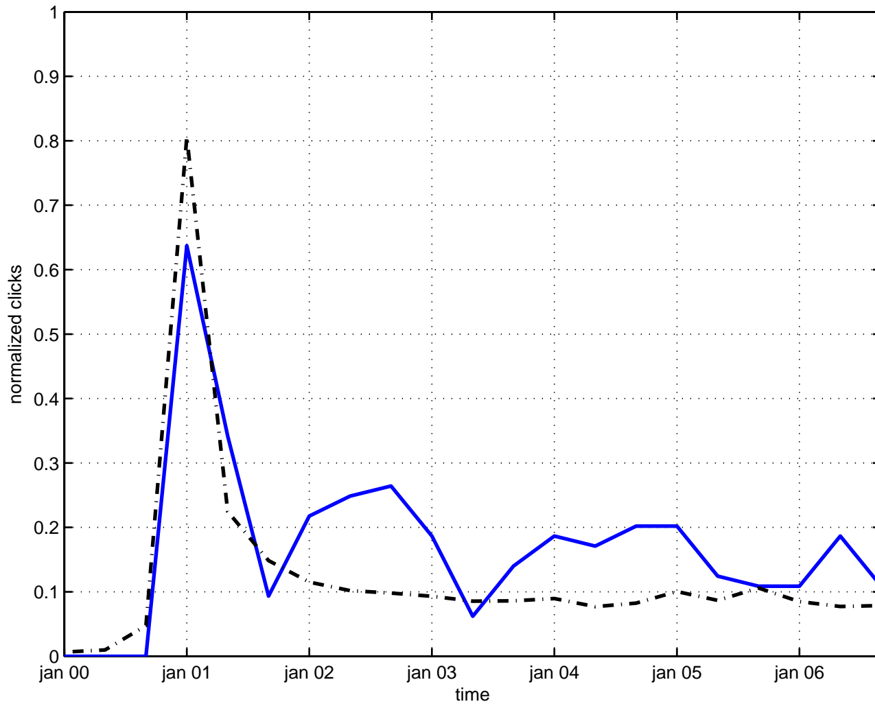
muonium
