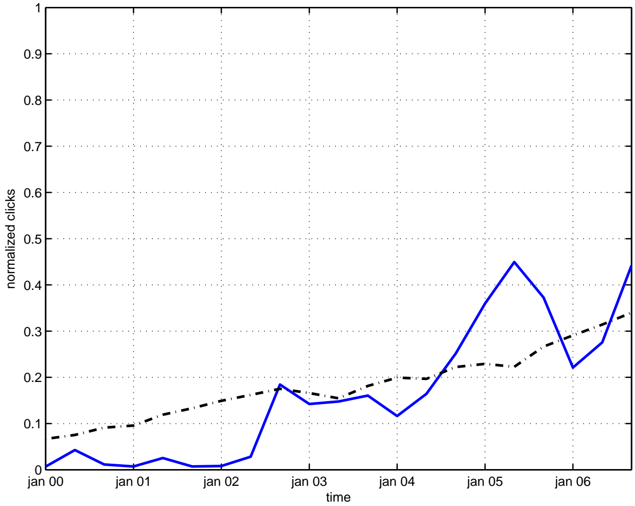
minisuperspace
