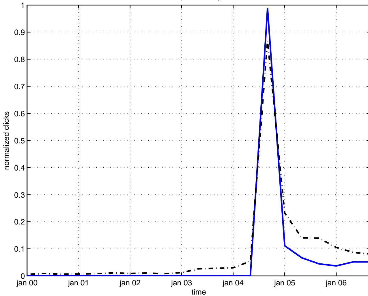
mass spectrum skyrmion
