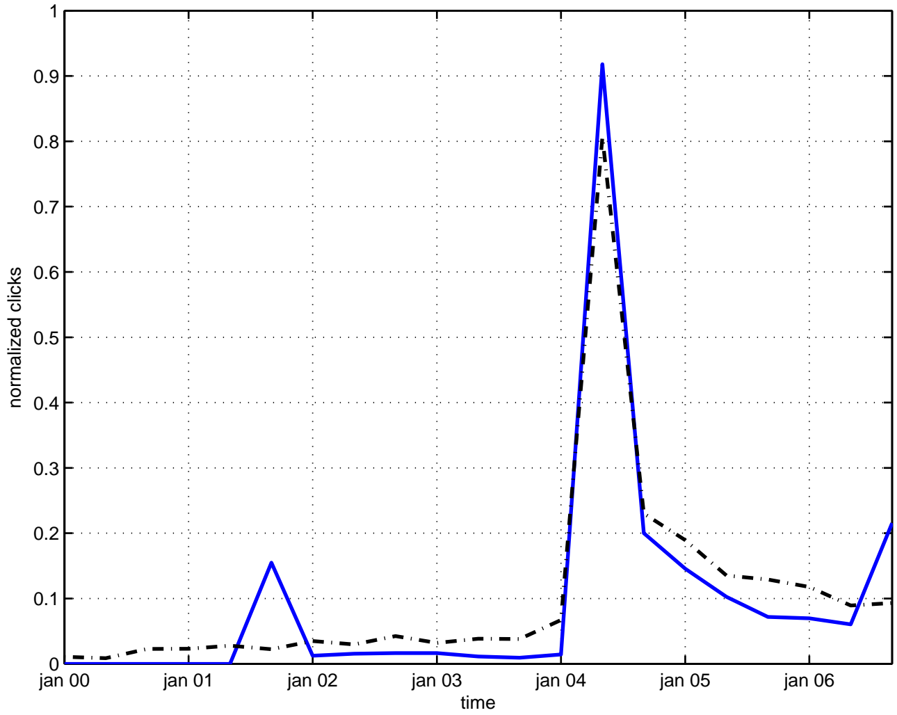
mass eta(958)
