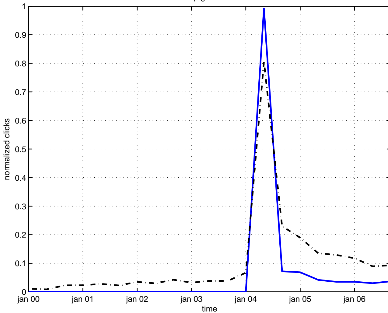
lsp gravitino
