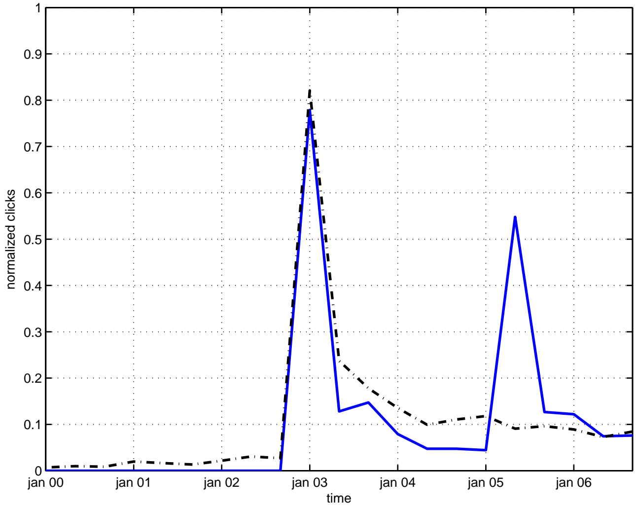
liouville gravitation
