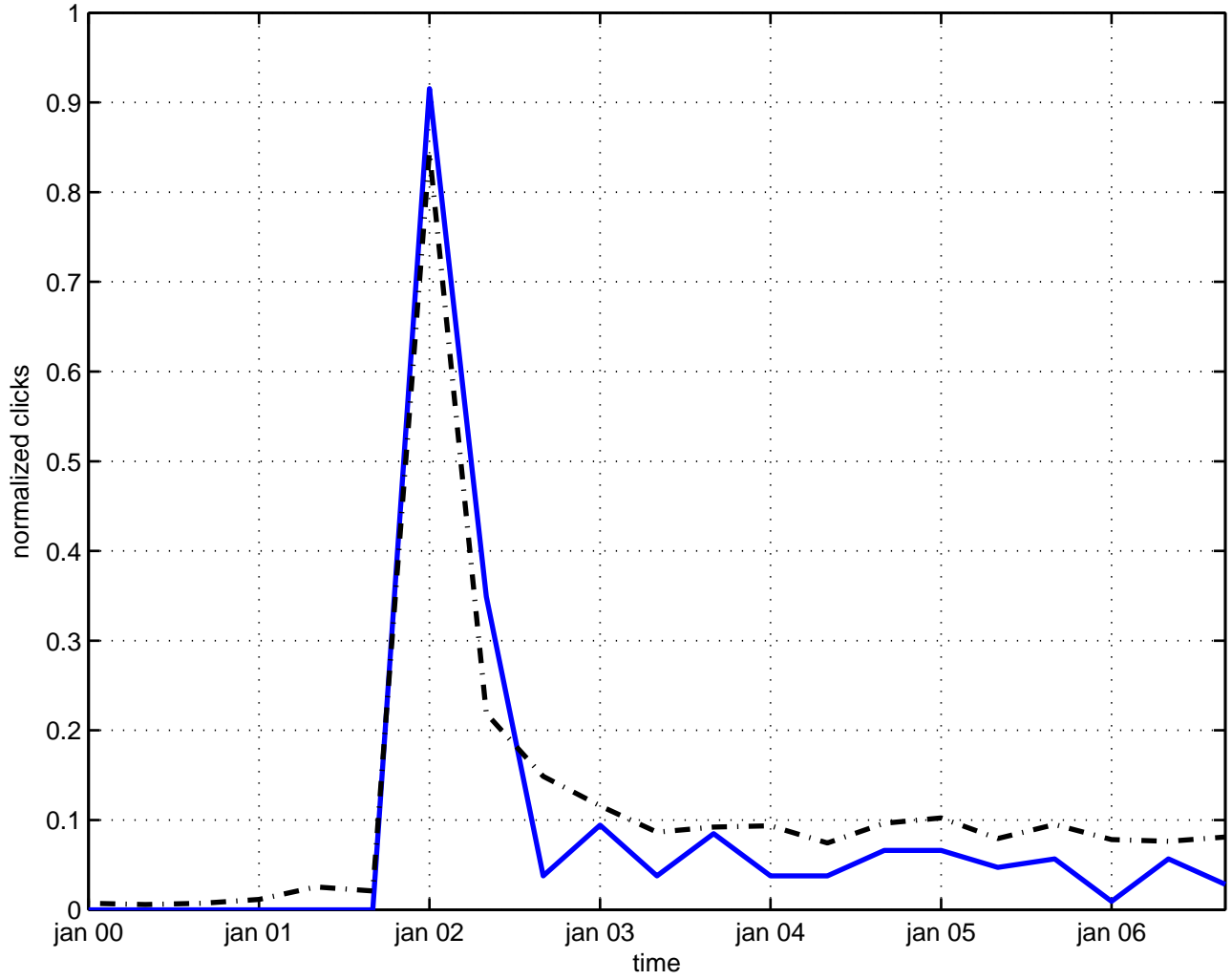
linear multiplet
