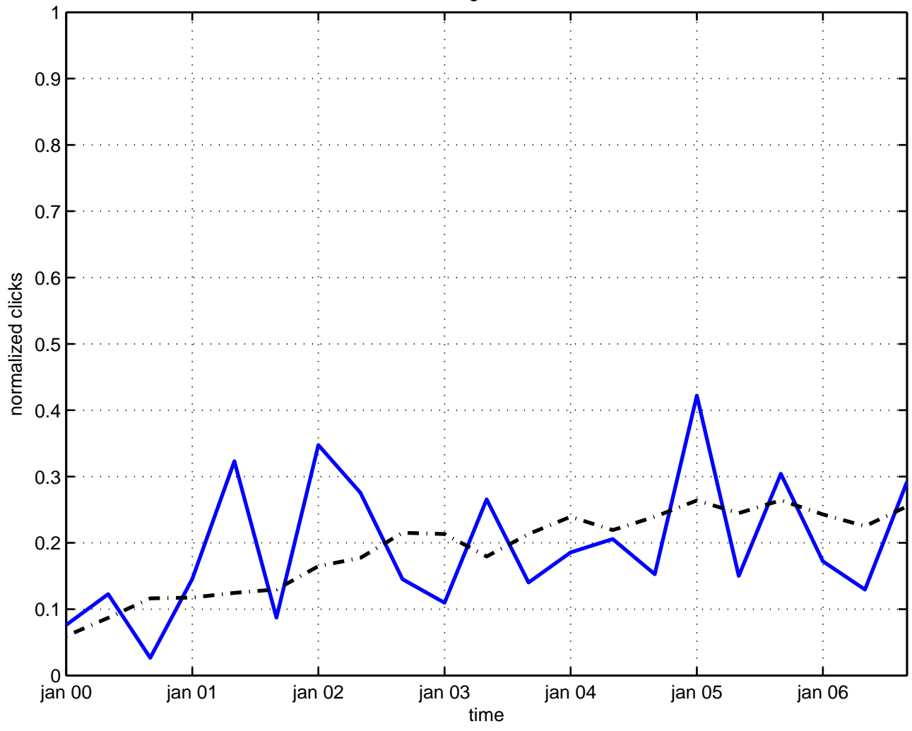
linear gravitation
