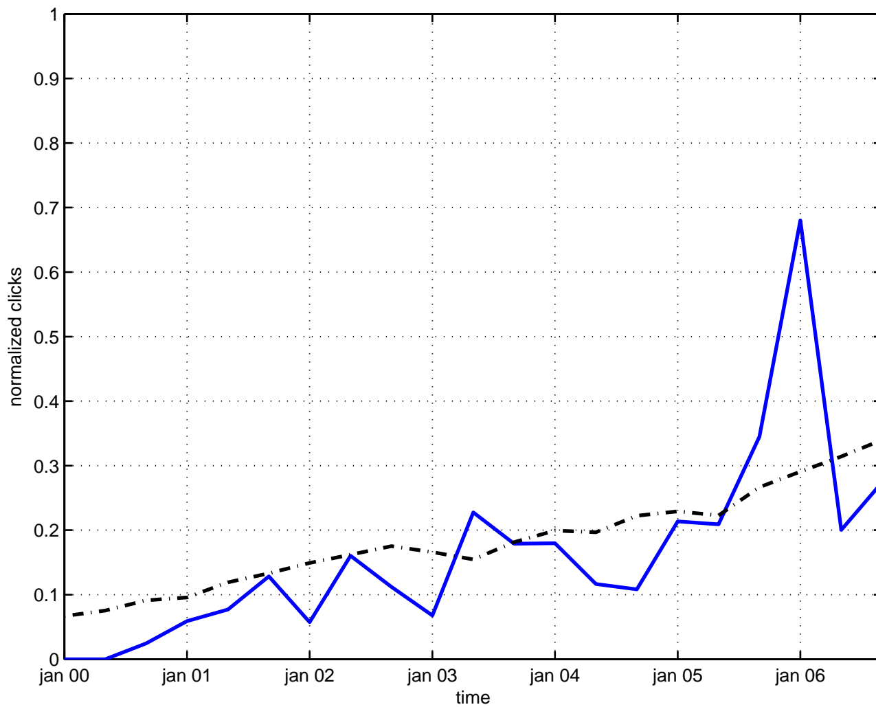
linear dilaton
