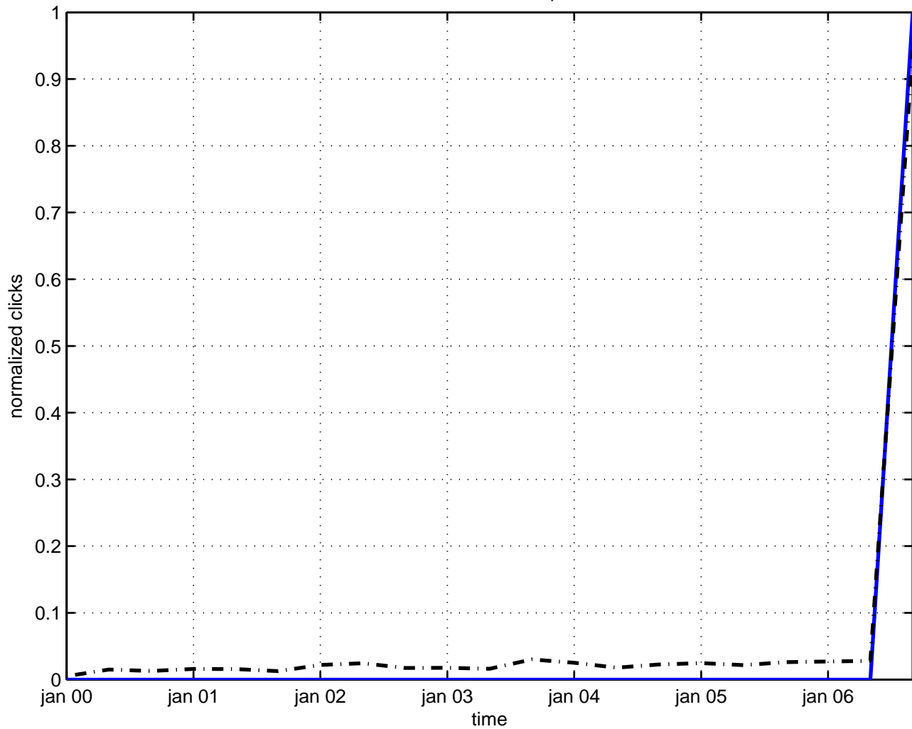
kaluza-klein monopole
