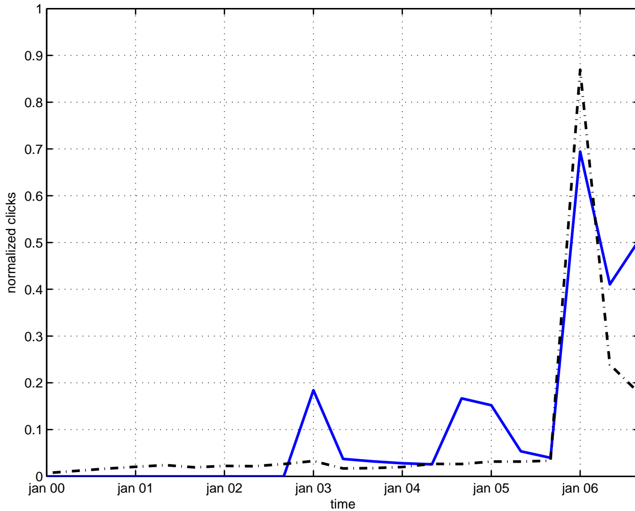
k-essence
