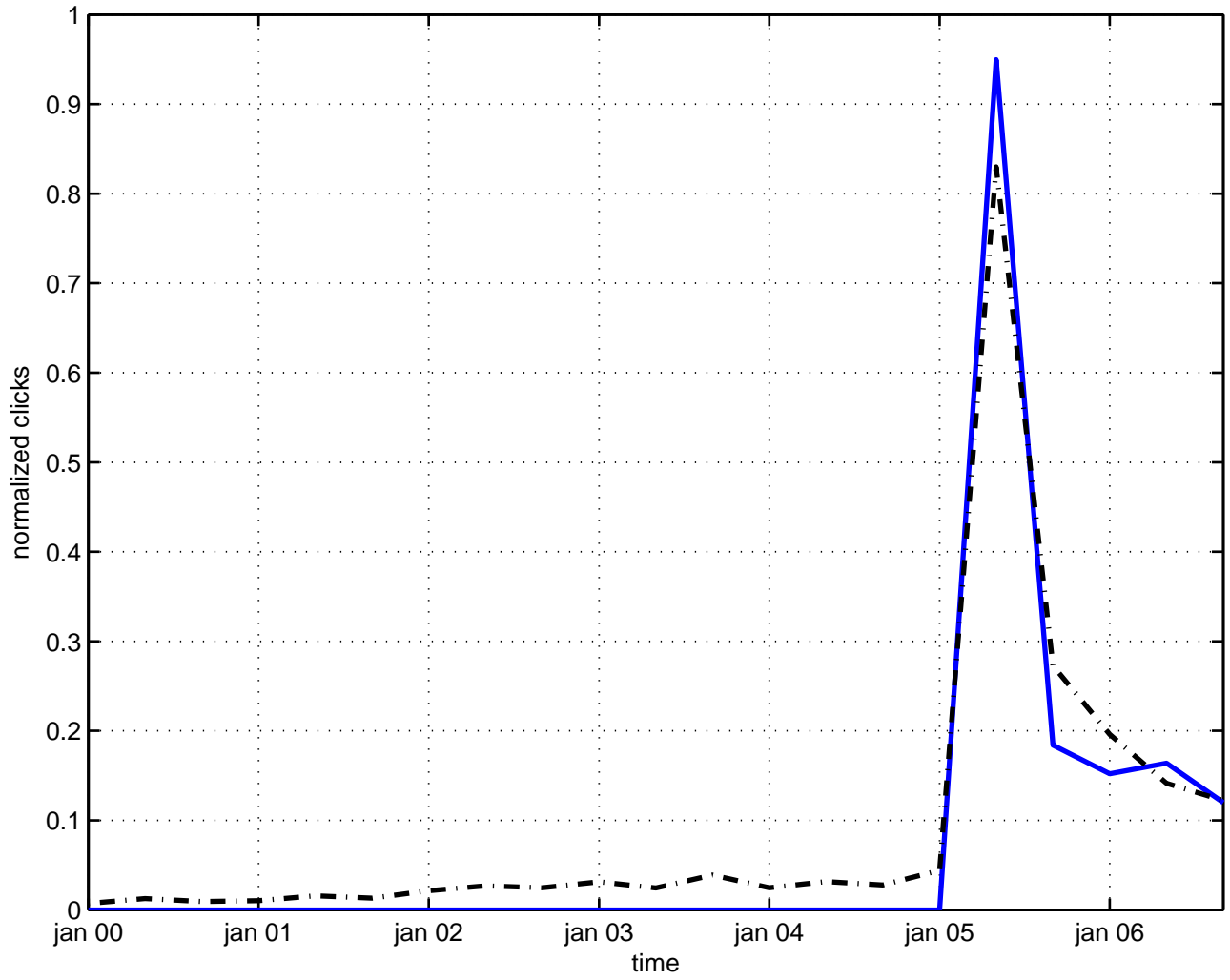
invariance reparametrization
