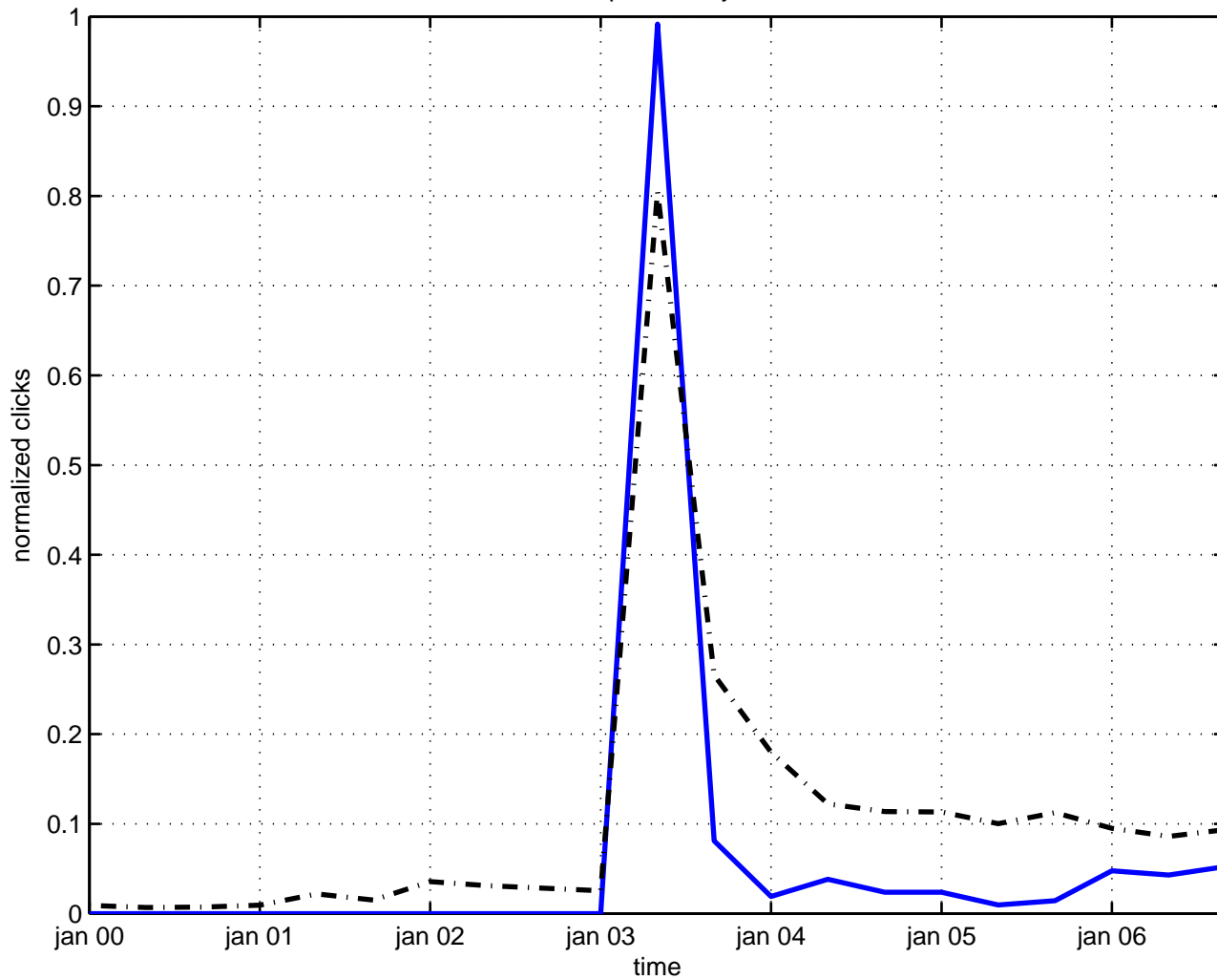
hopf anomaly
