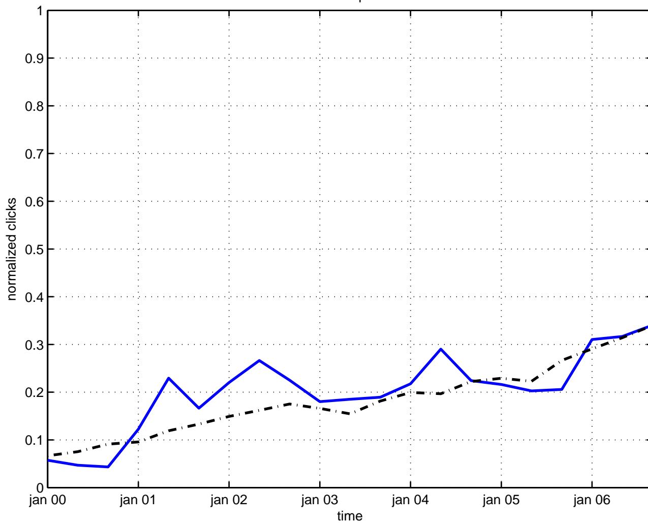
hilbert space
