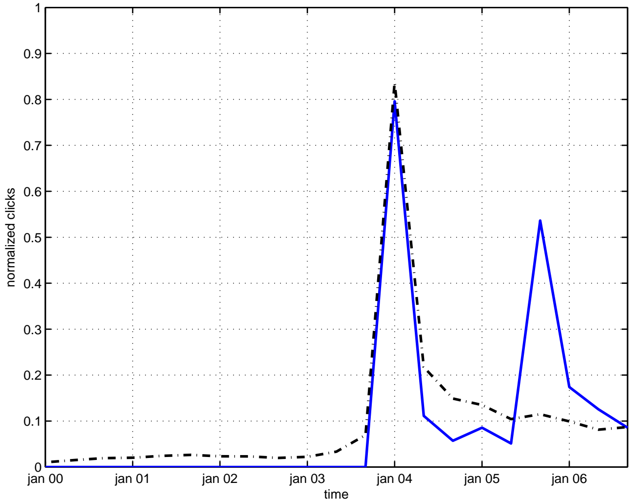
hierarchy soliton
