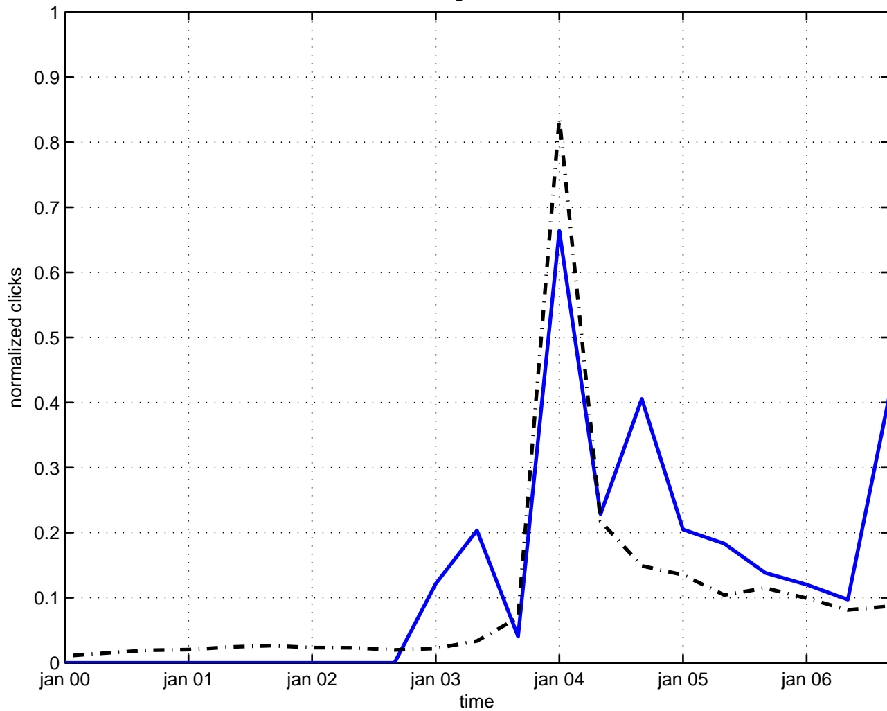
gluon
