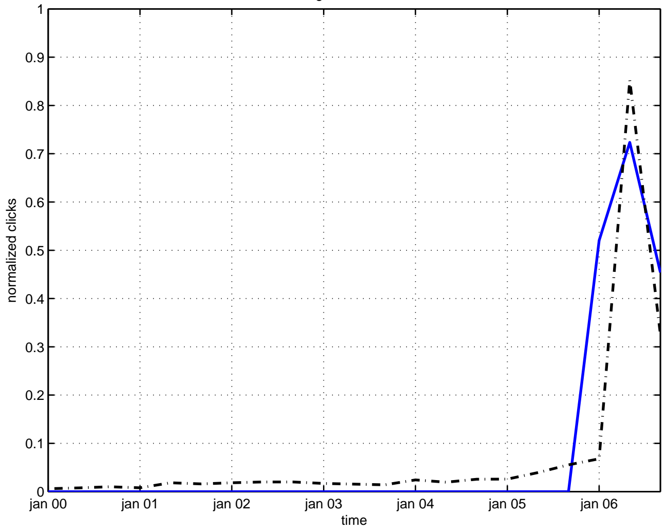
global vortex
