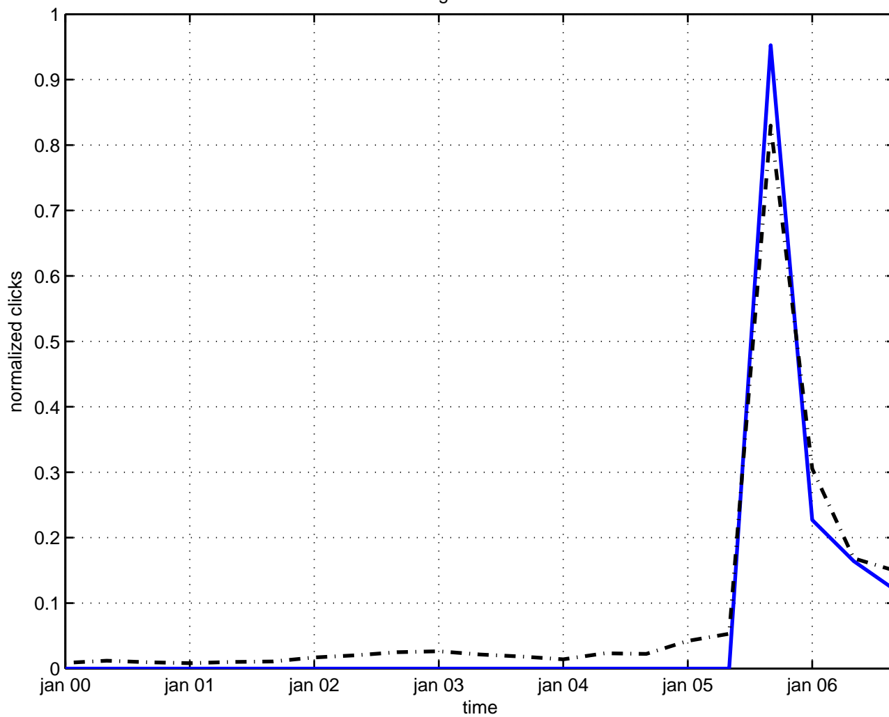
geodesics
