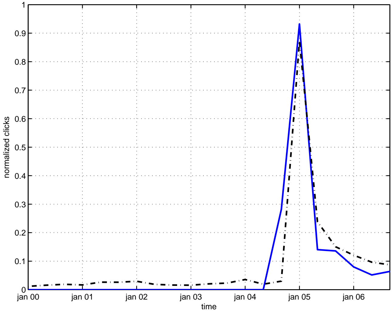
froissart bound
