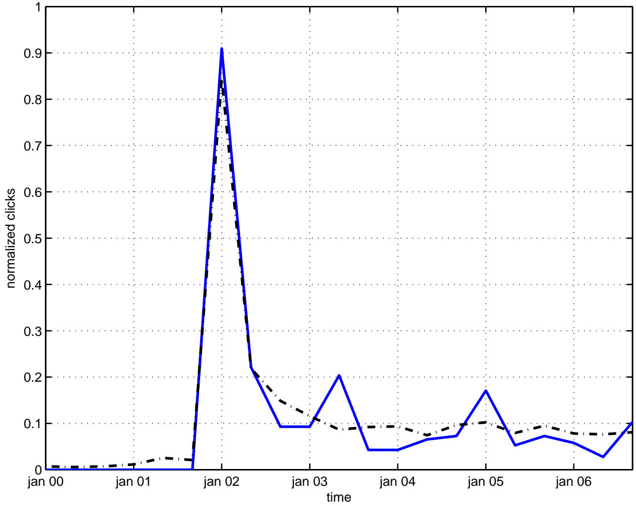
froissart bound cross section
