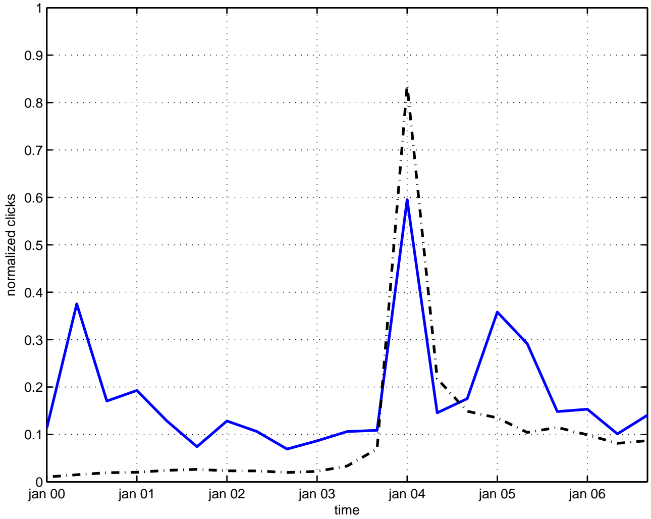
feynman gauge
