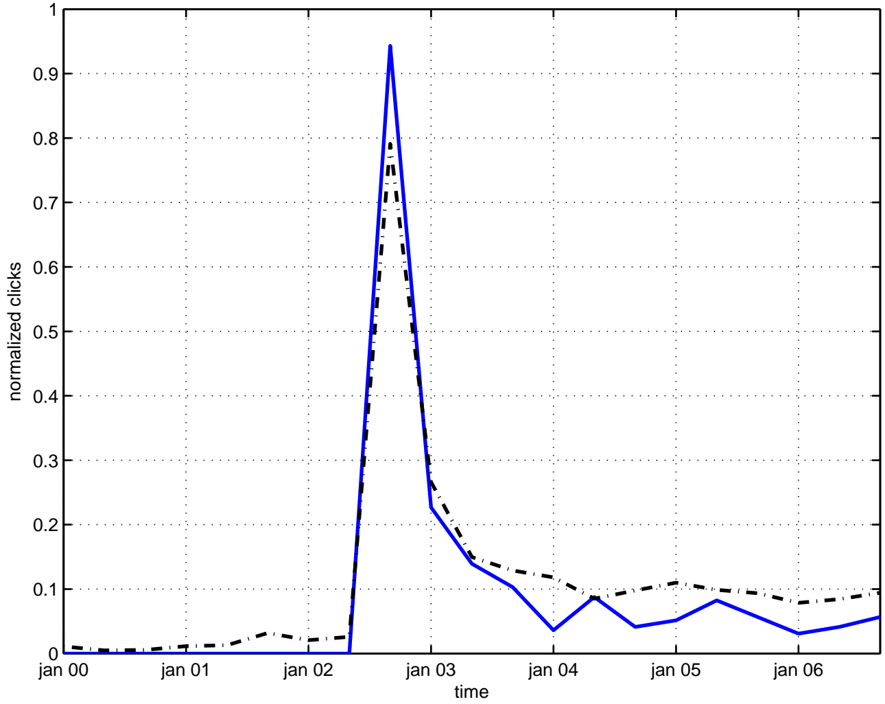
ferromagnet string
