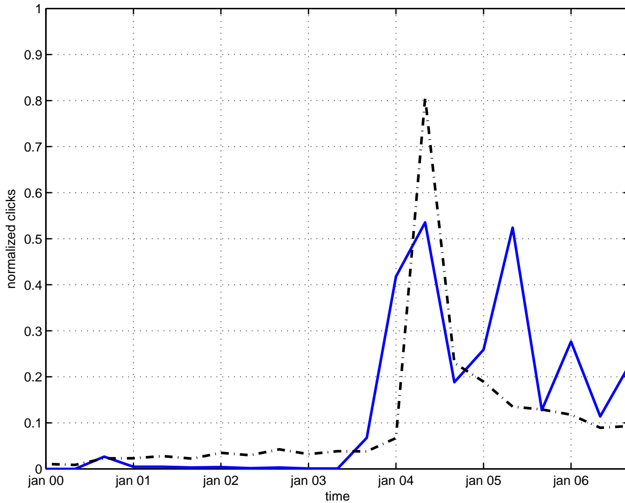
fermionization
