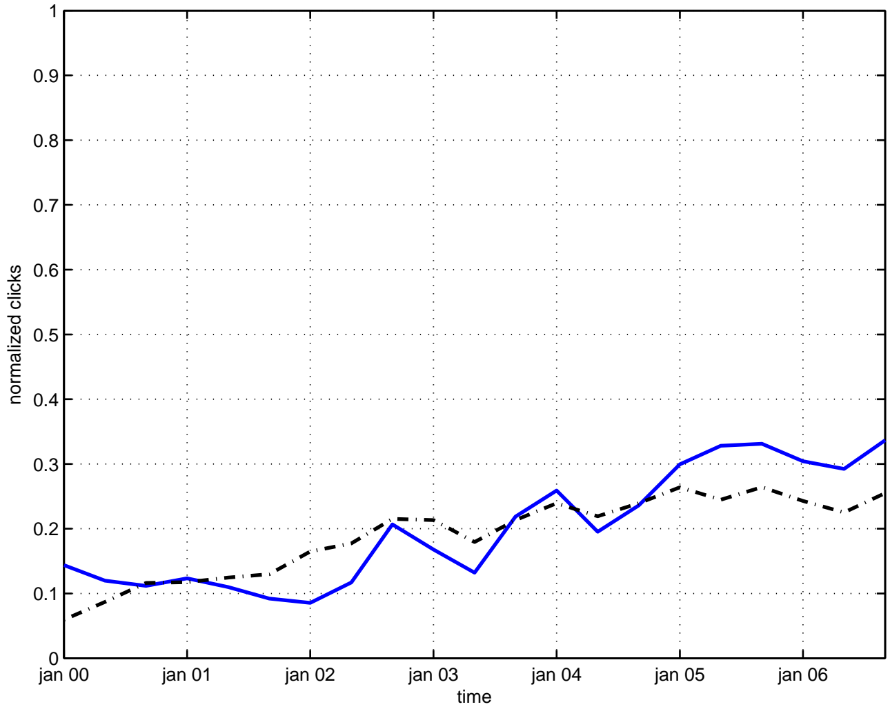
fermion
