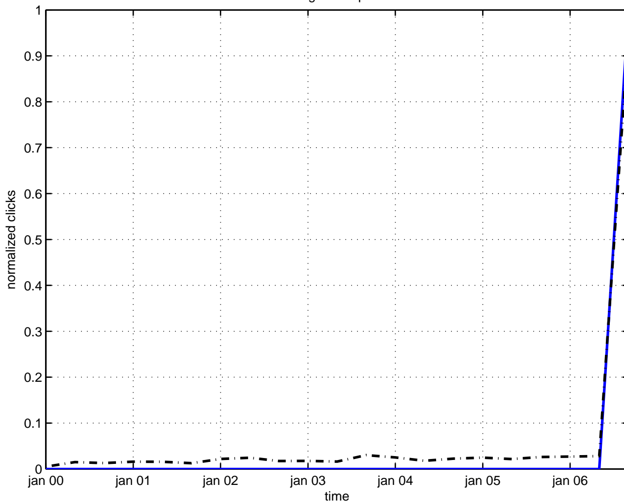
entanglement photon
