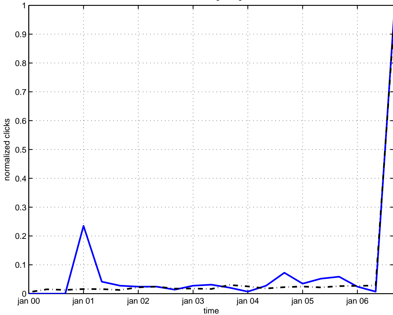
embedding string
