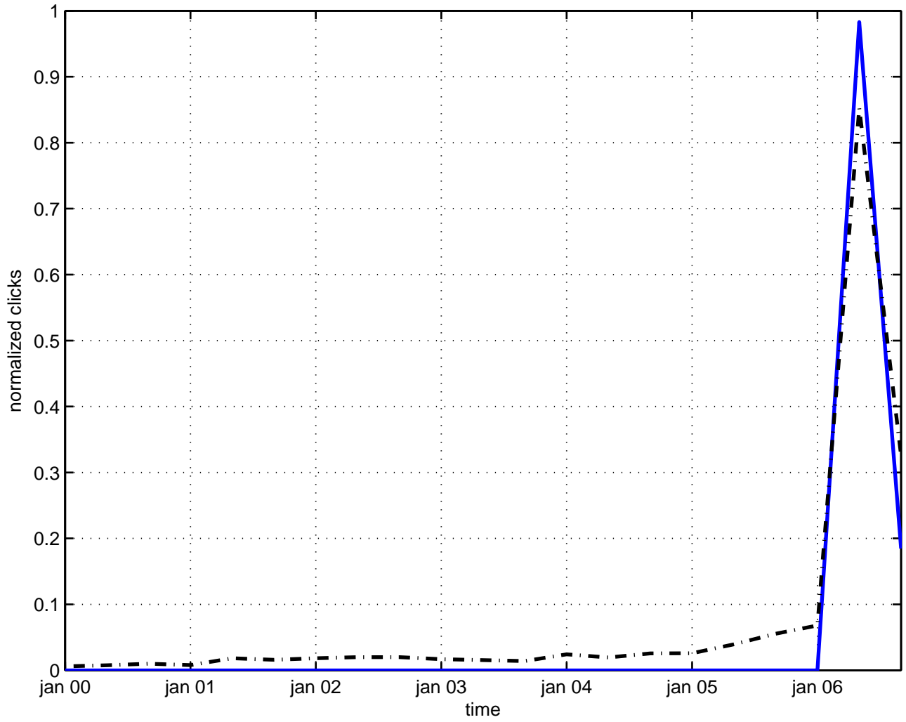
droplet bosonization
