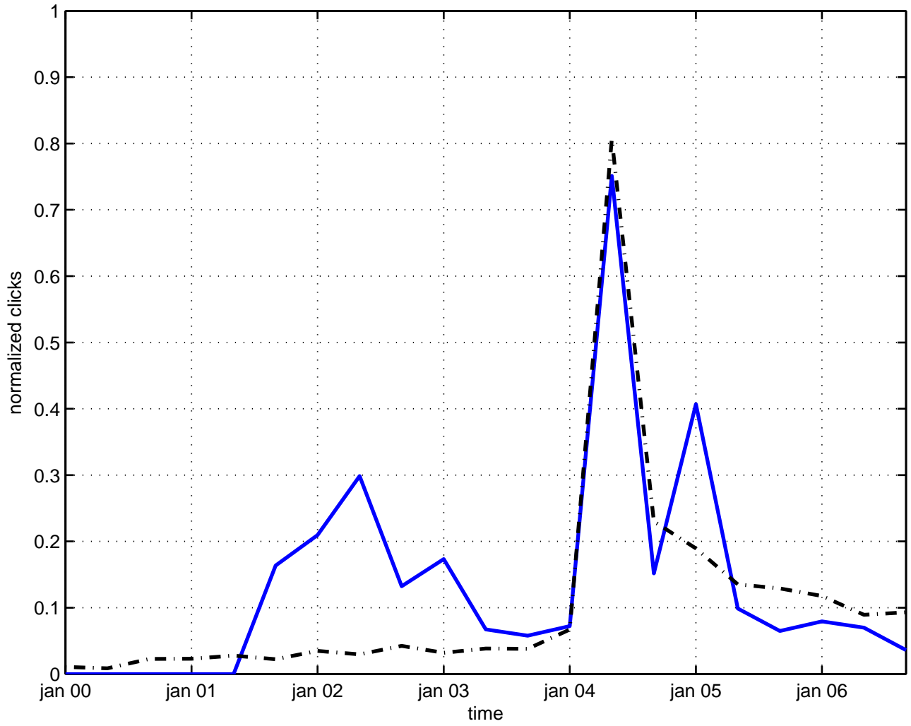
dirac neutrino
