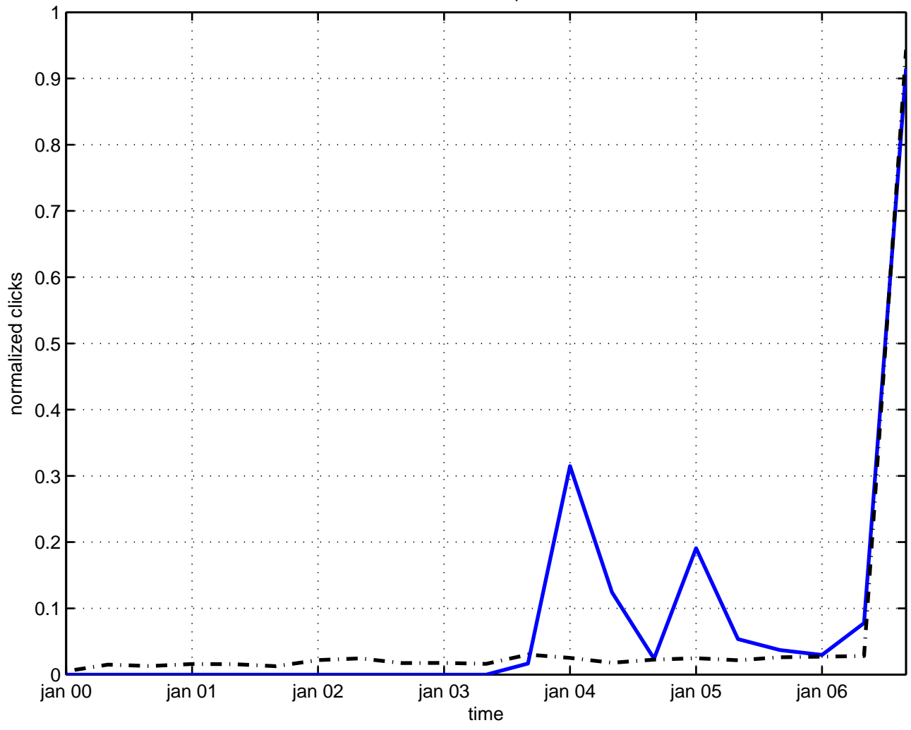
dirac monopole
