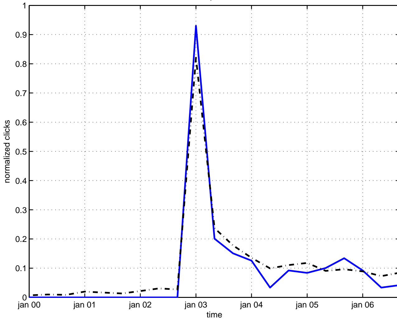
diquark
