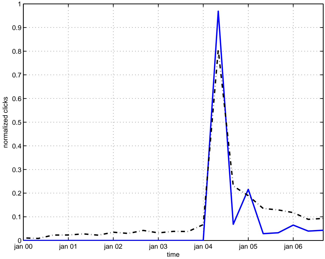
decay sphaleron
