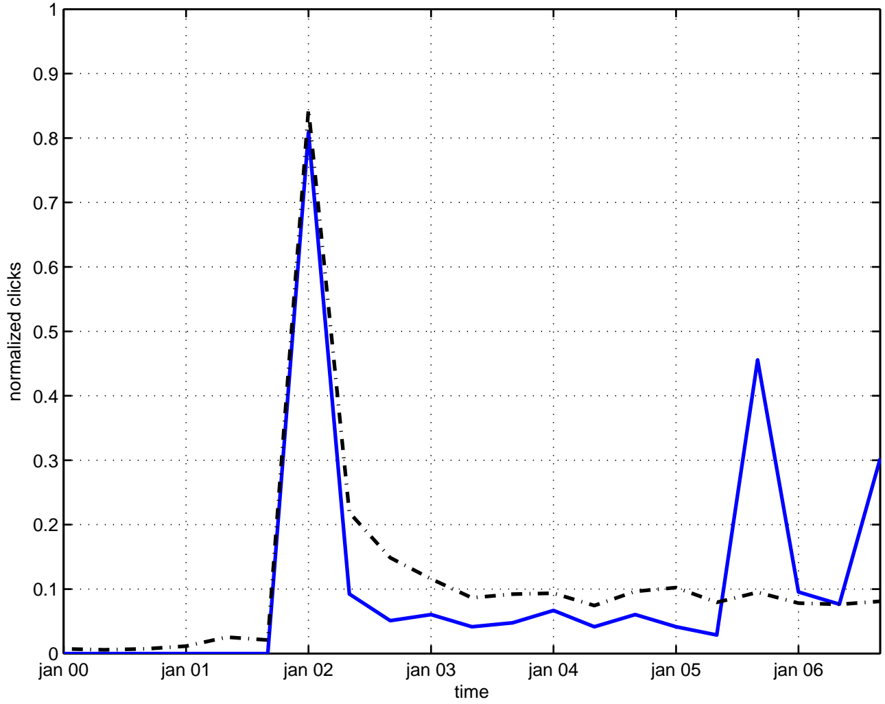
de sitter background
