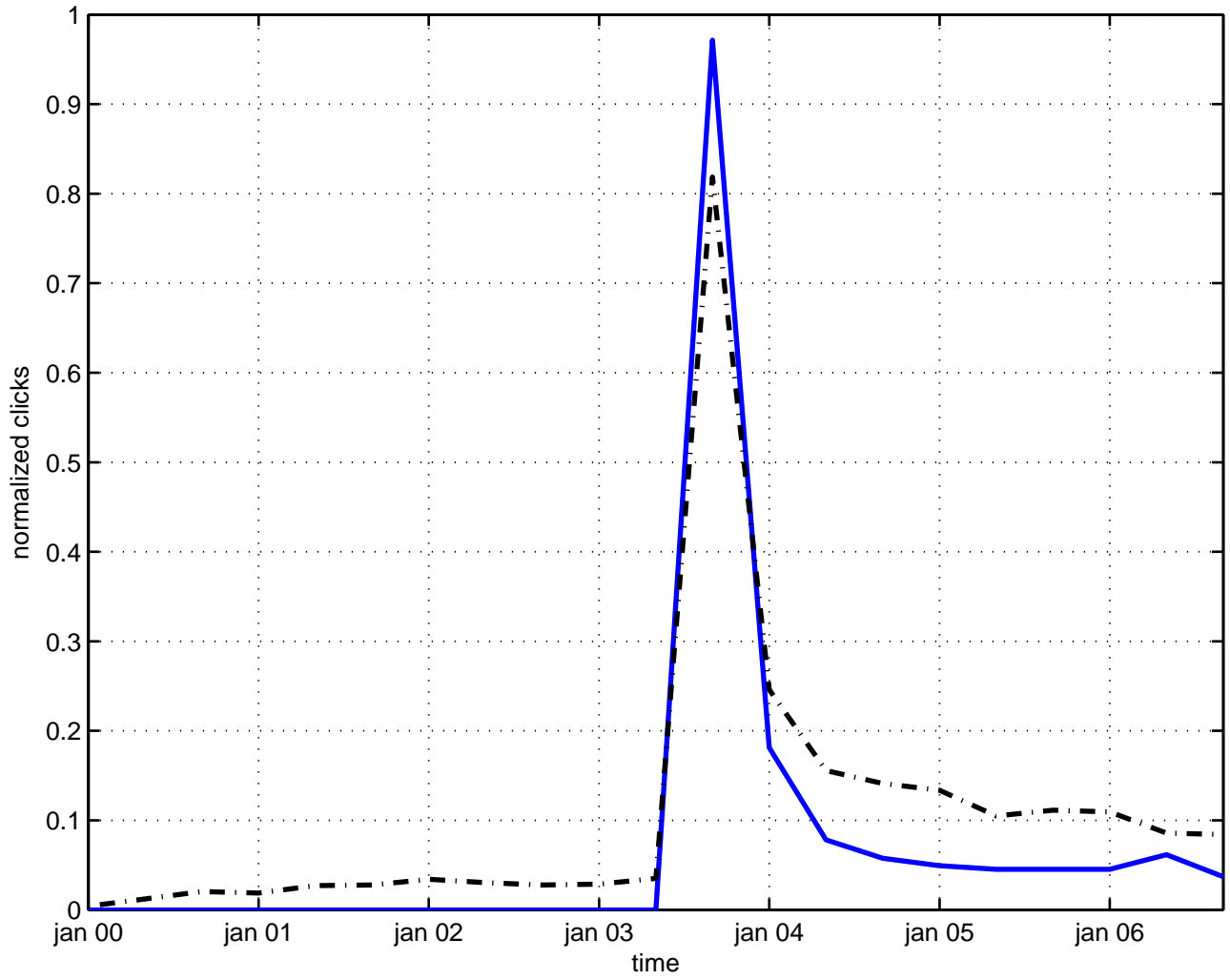
d-brane membrane
