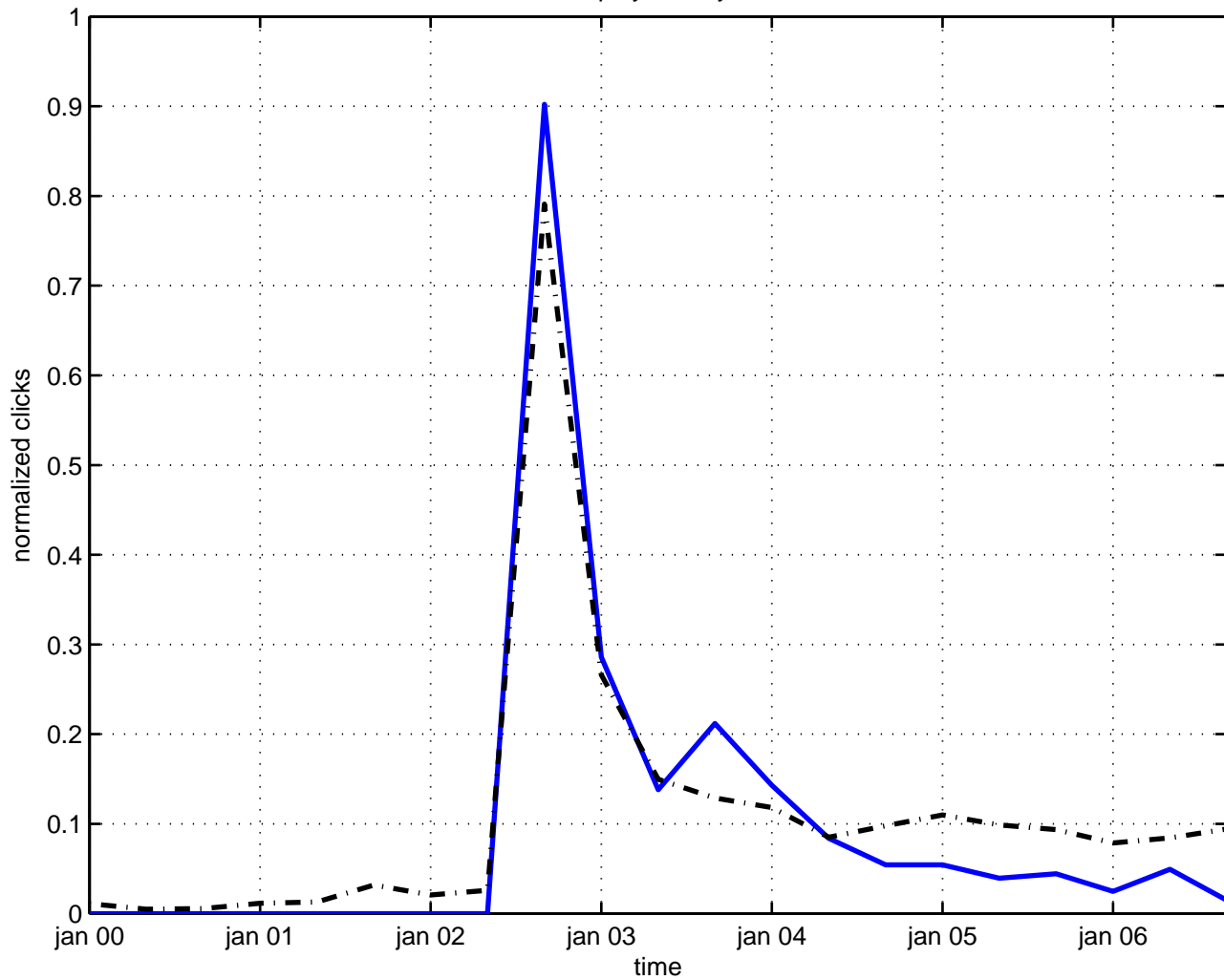
cp symmetry
