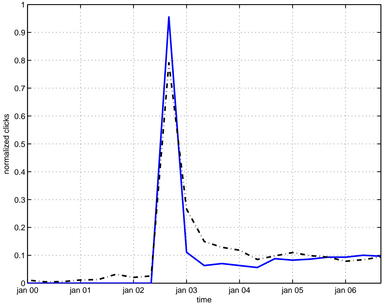
cp invariance
