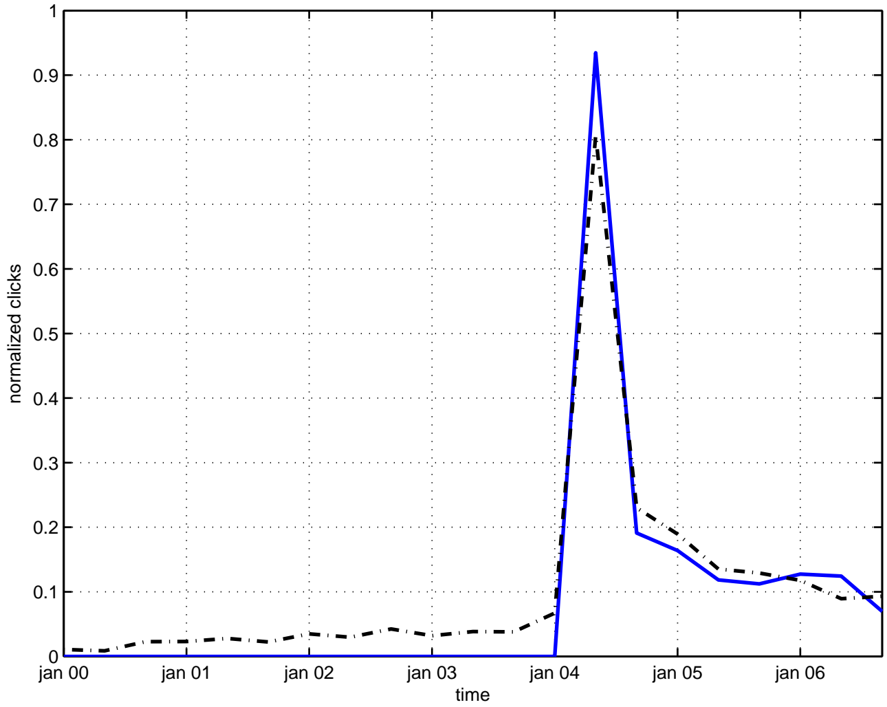
cp(n-1) quantum space
