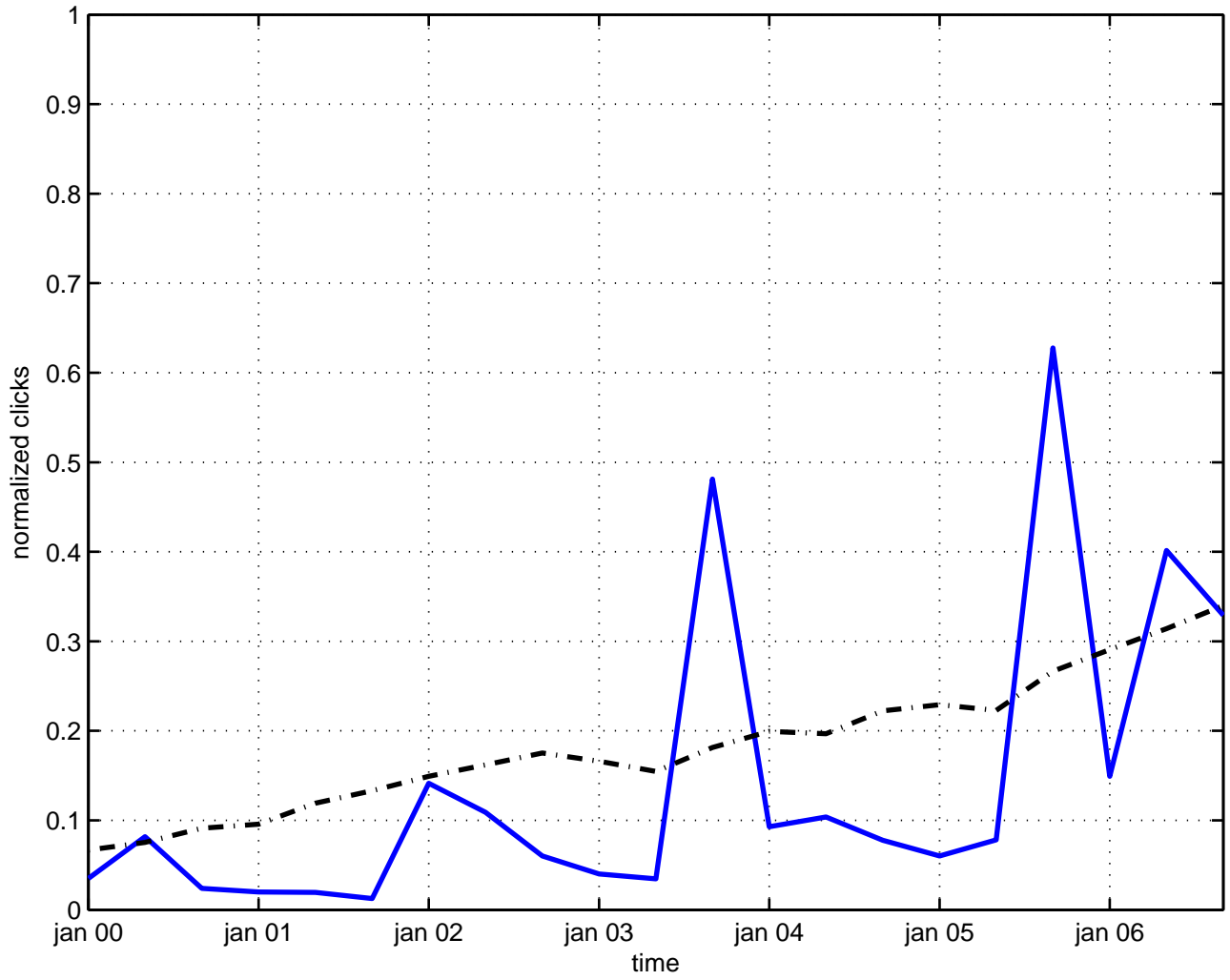
cp(n) space
