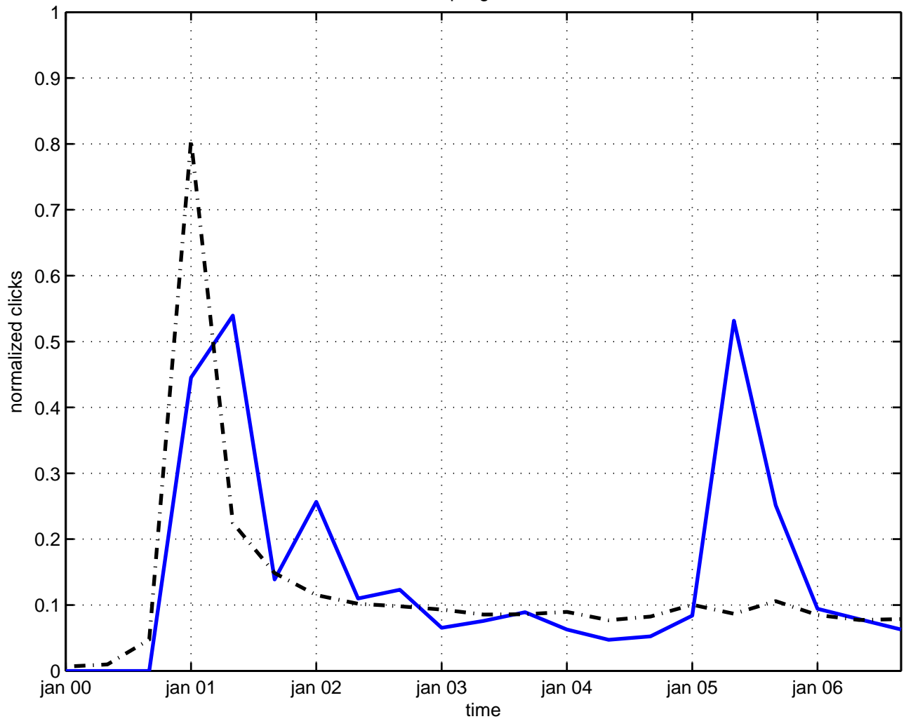
coupling radion
