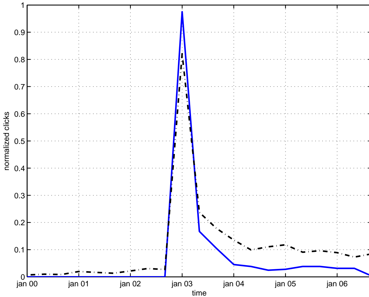
confinement ion
