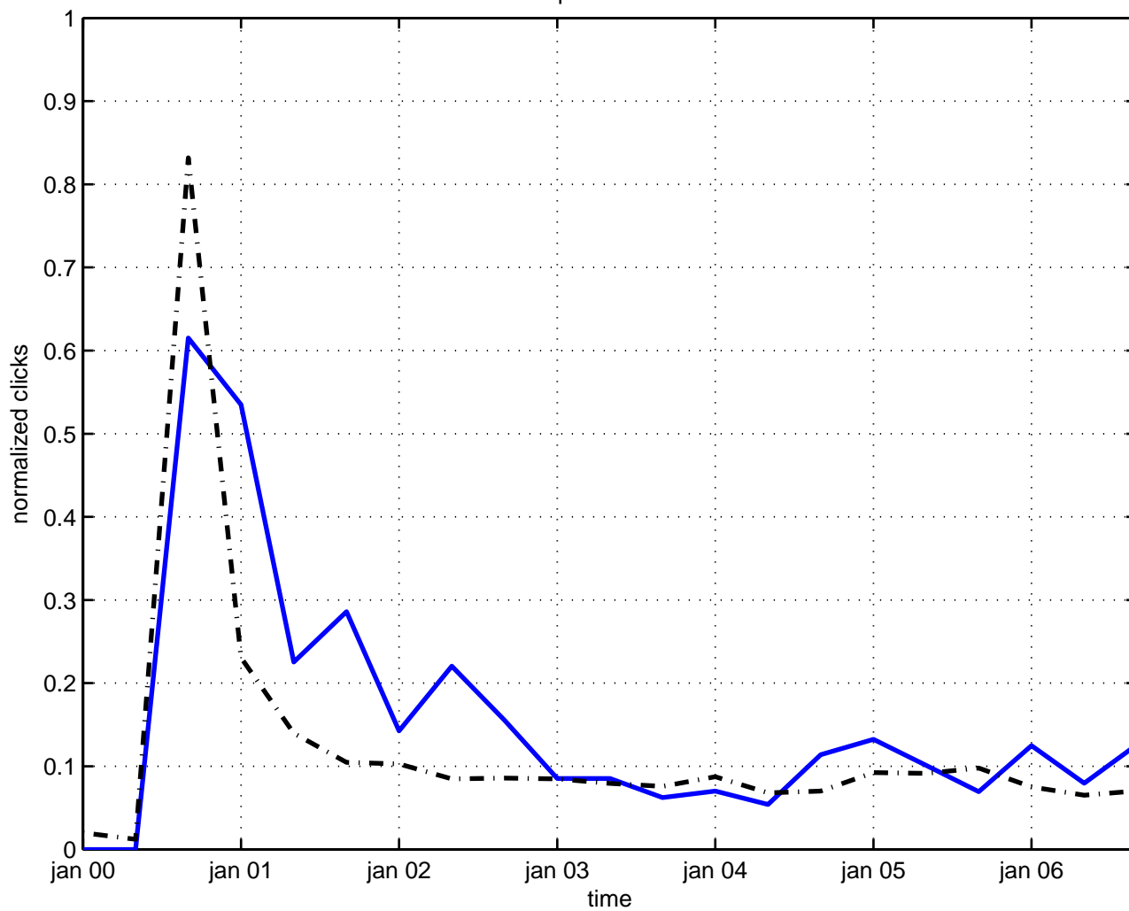
composite fermion
