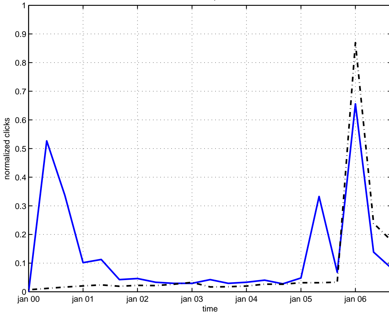
circle space
