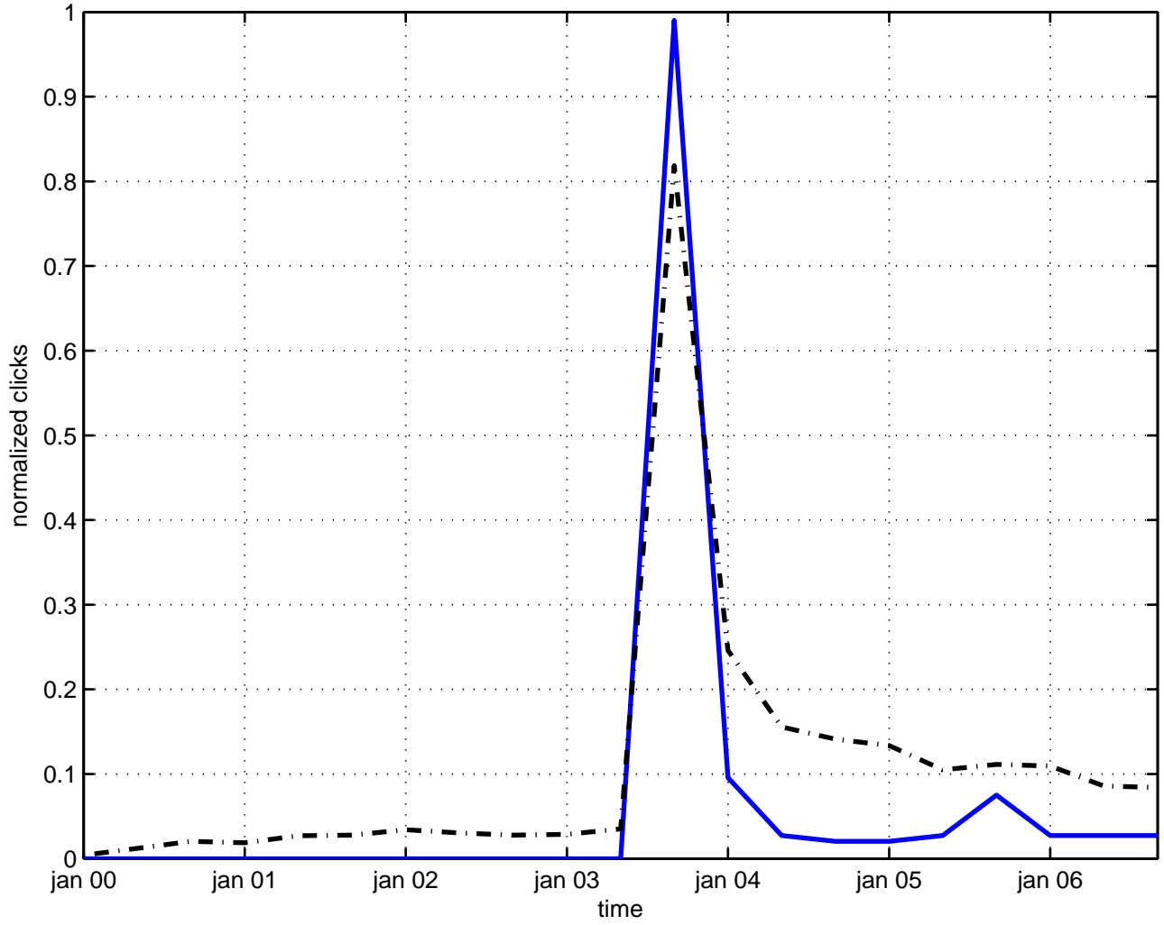
charge fermion
