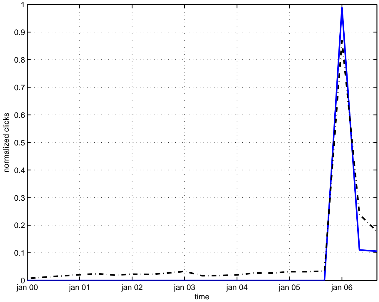
c(n)/z(m) space
