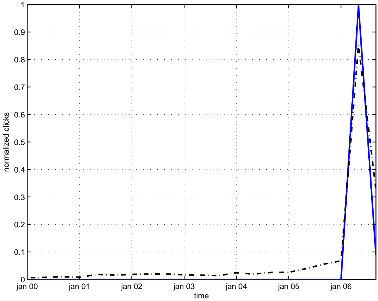
c(3)/z(6) space
