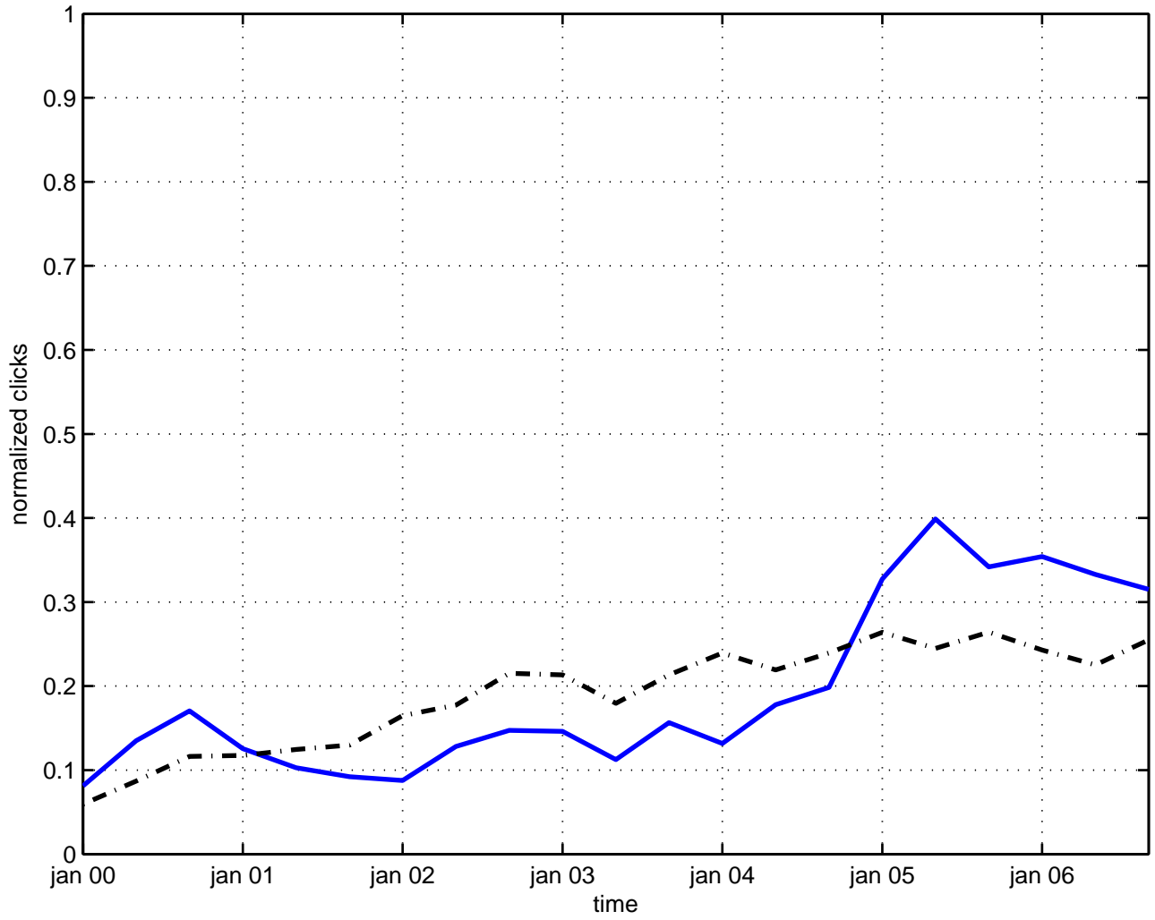
bps soliton
