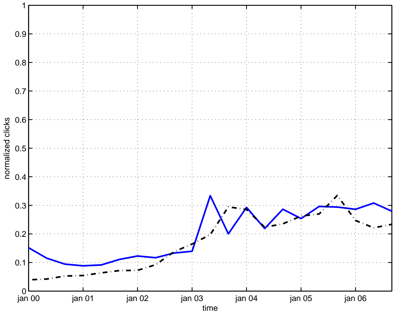
bosonization
